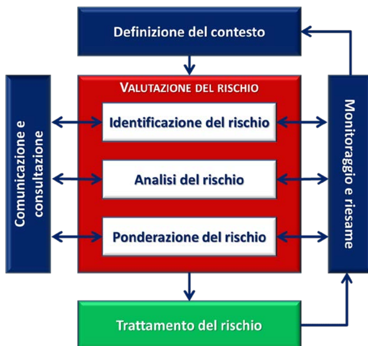
Figura 10 - ISO 31000 (2009)
