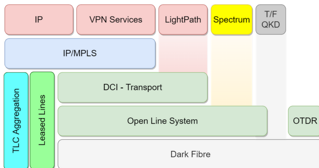
Figura 6: Architettura di rete GARR-T
